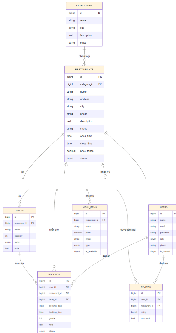
Hình 2.2: Sơ đồ thực thể - liên kết (ERD) của hệ thống cơ sở dữ liệu
